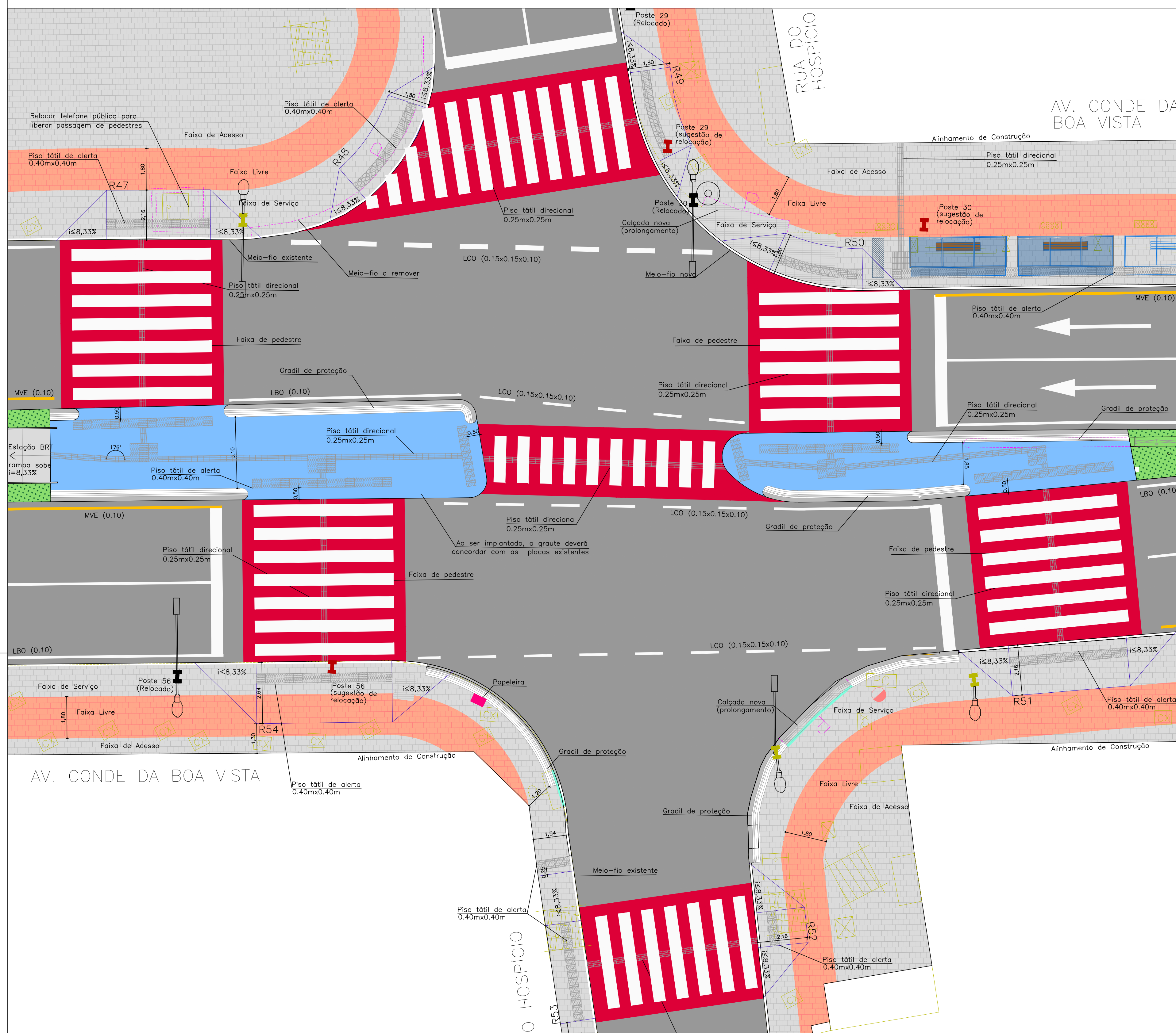
INTERSEÇÃO 08 - AV. CONDE DA BOA VISTA x RUA DO HOSPÍCIO ESC. 1/100
