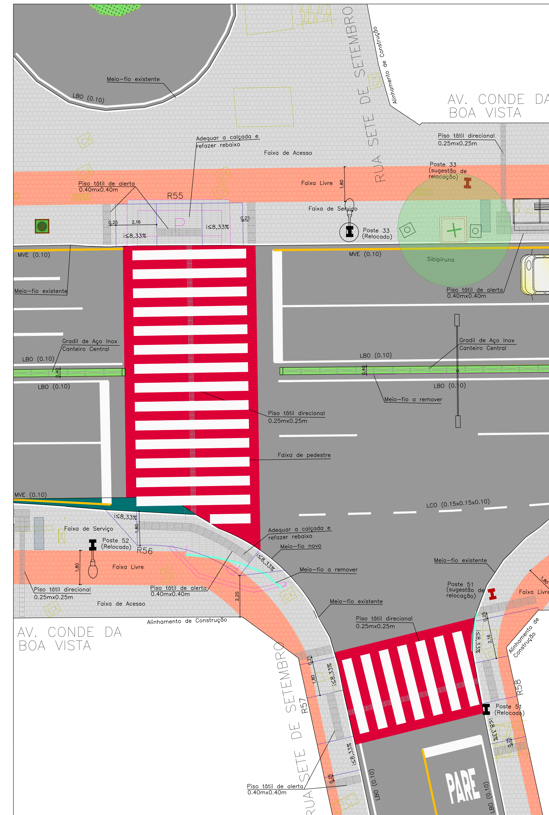
INTERSEÇÃO 09 - AV. CONDE DA BOA VISTA x RUA SETE DE SETEMBRO ESC. 1/100
