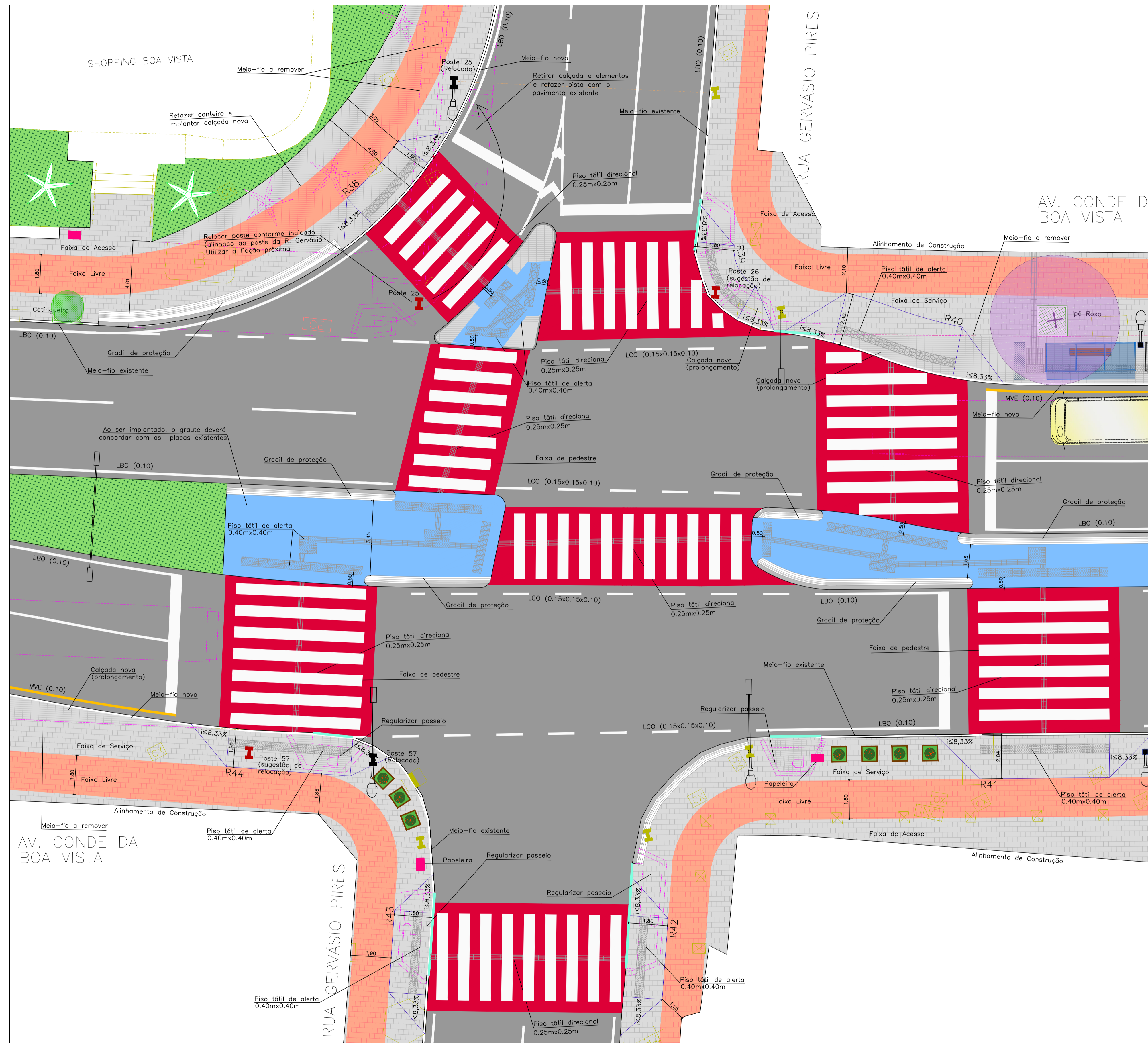
INTERSEÇÃO 07 - AV. CONDE DA BOA VISTA x RUA GERVÁSIO PIRES ESC. 1/100
