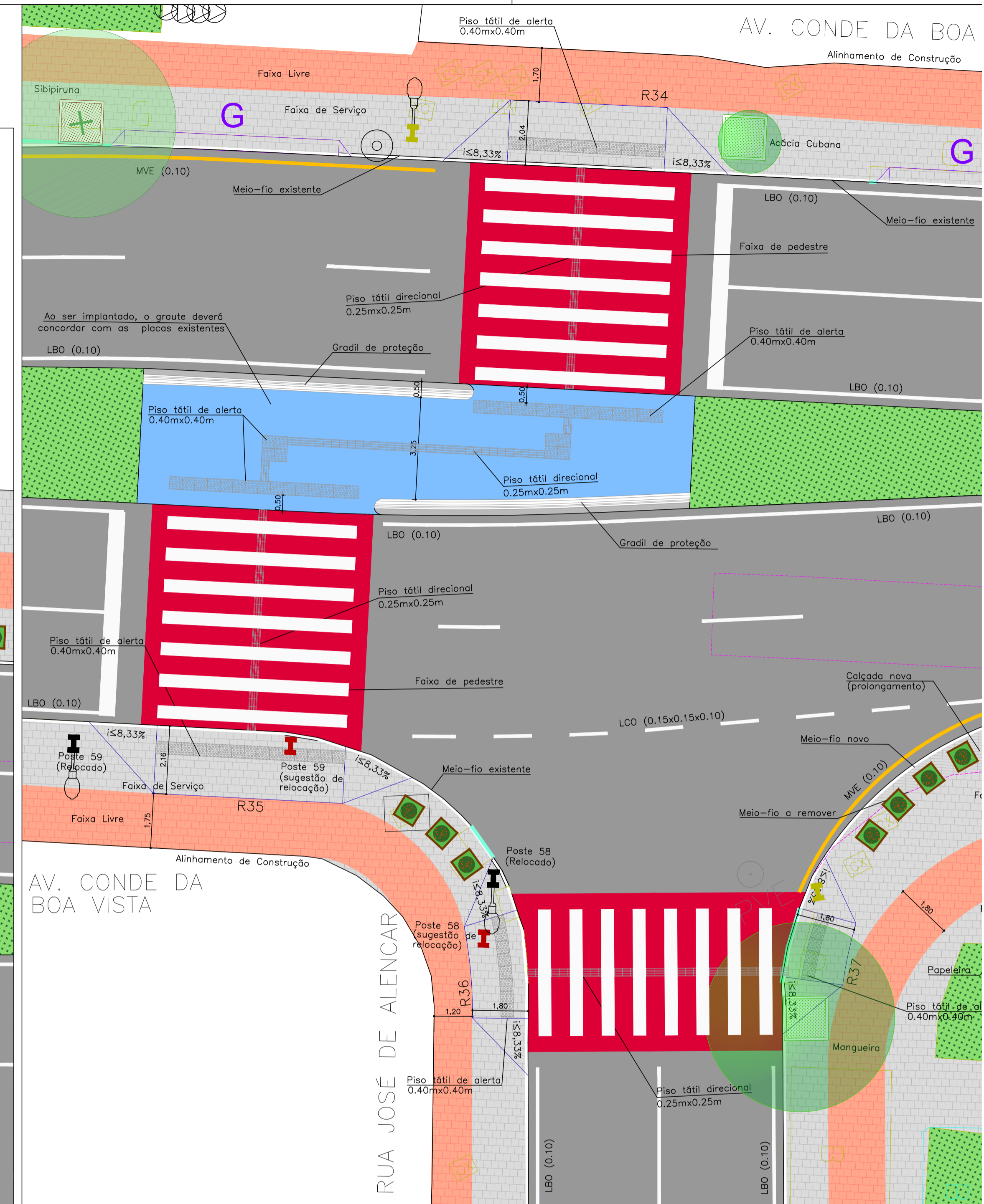
INTERSEÇÃO 06 - AV. CONDE DA BOA VISTA x RUA JOSÉ DE ALENCAR ESC. 1/100
