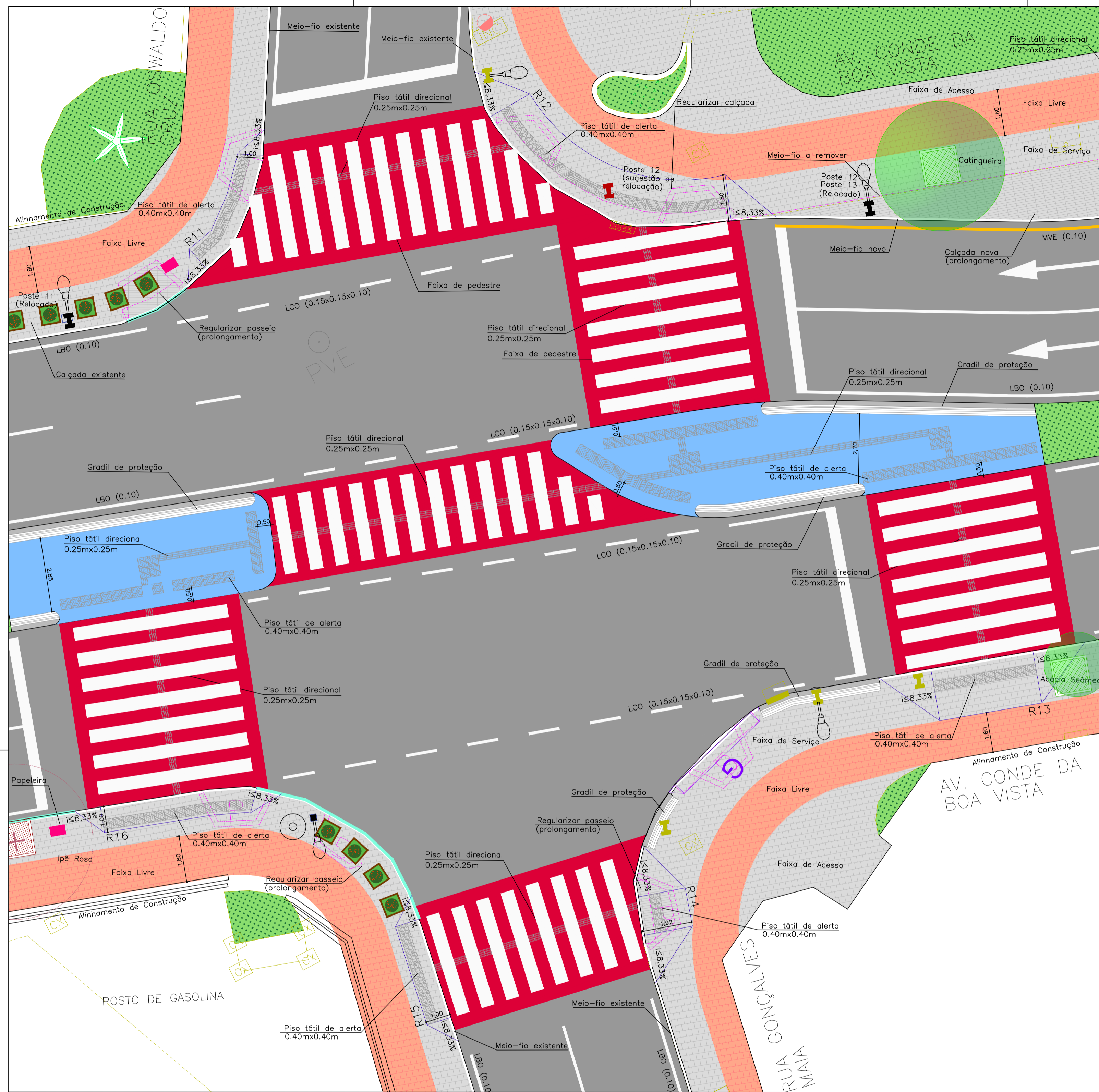
INTERSEÇÃO 03 - AV. CONDE DA BOA VISTA x RUA OSWALDO CRUZ/RUA GONÇALVES MAIA ESC. 1/100
