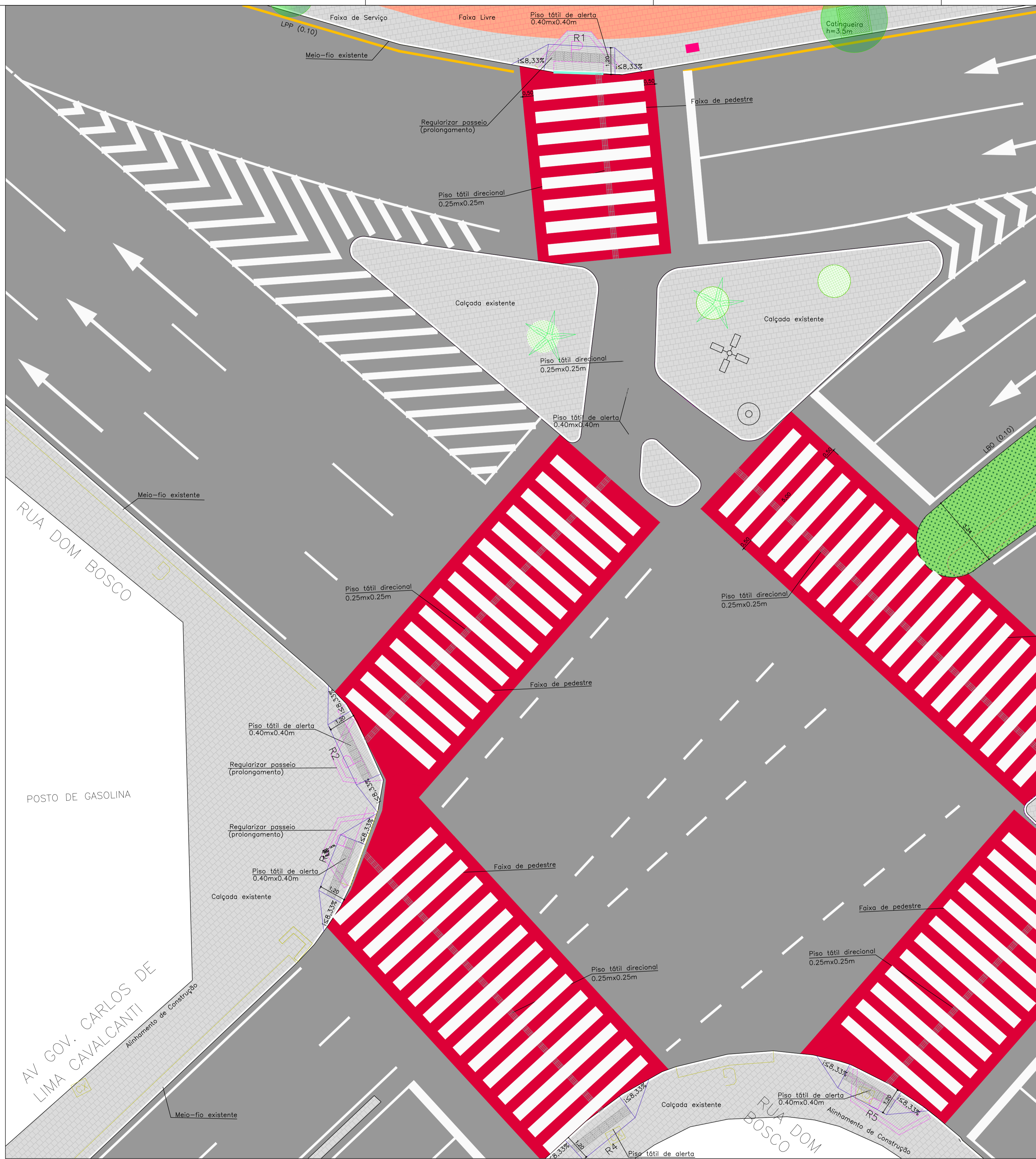
INTERSEÇÃO 01 - AV. CONDE DA BOA VISTA x RUA DOM BOSCO ESC. 1/100
