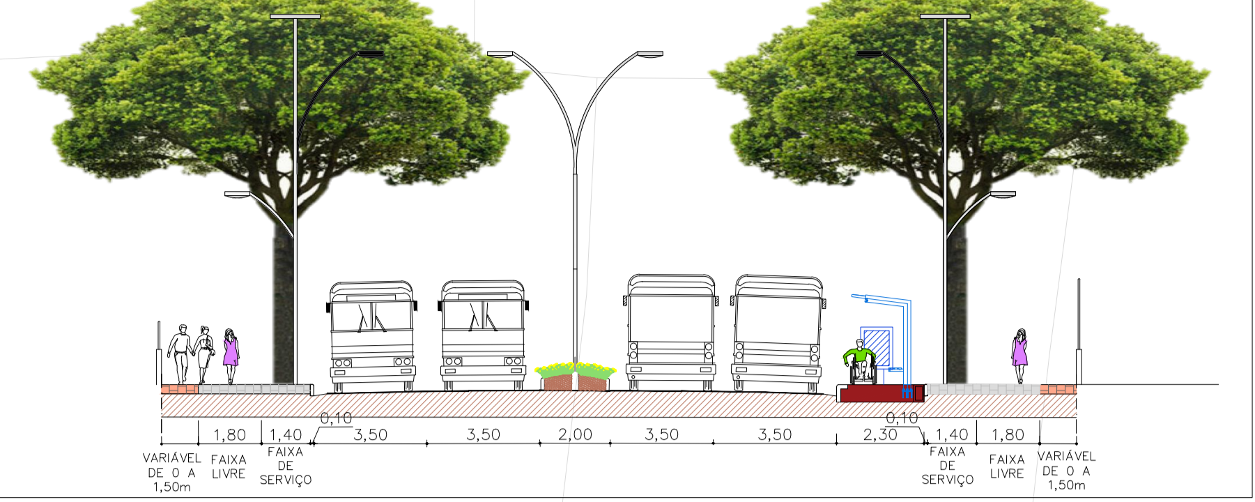
SEÇÃO AA
